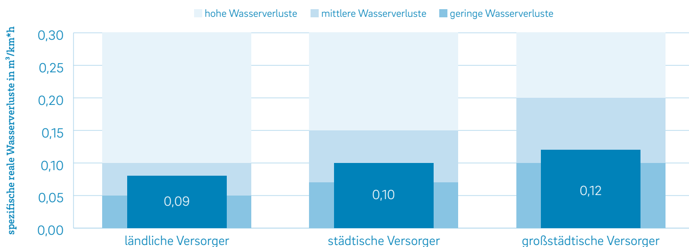
Abbildung 11: mittlere spezifische reale Verluste in \text{m}^3/(\text{km}\cdot\text{h}) nach Urbanitätsgrad
