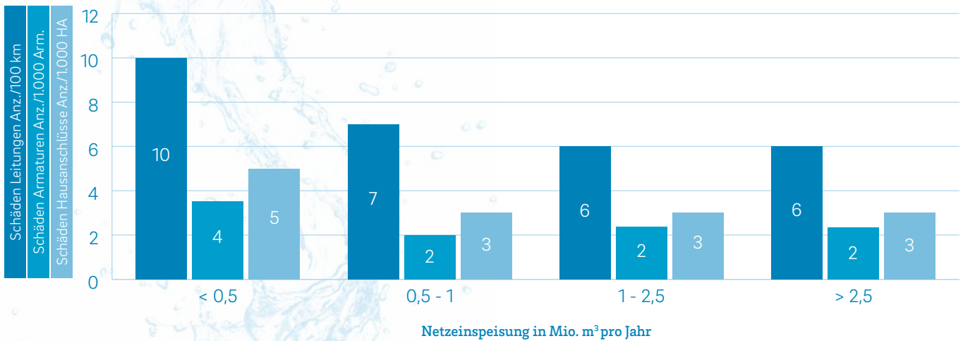
Abbildung 10: Gegenüberstellung Schadensraten Leitungen, Armaturen und Hausanschlüsse
